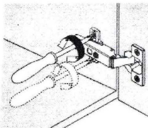
Reglare înălțime
